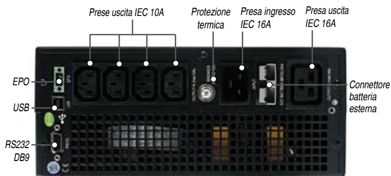
Sigma 3000 VA (vista posteriore)
