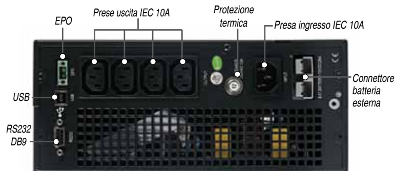
Sigma 2000 VA (vista posteriore)
