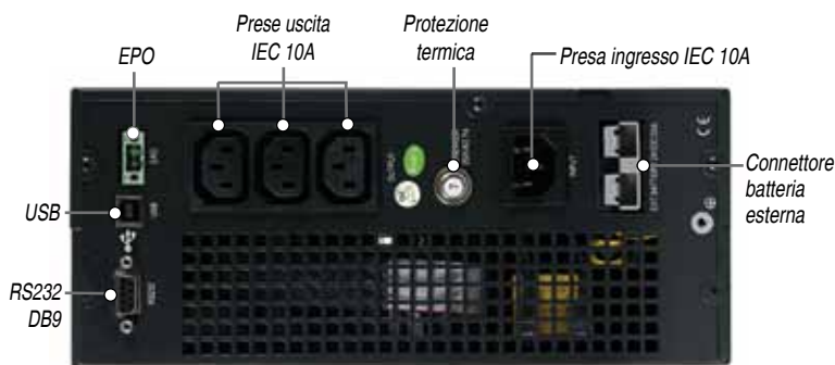
Sigma 1000 VA (vista posteriore)
